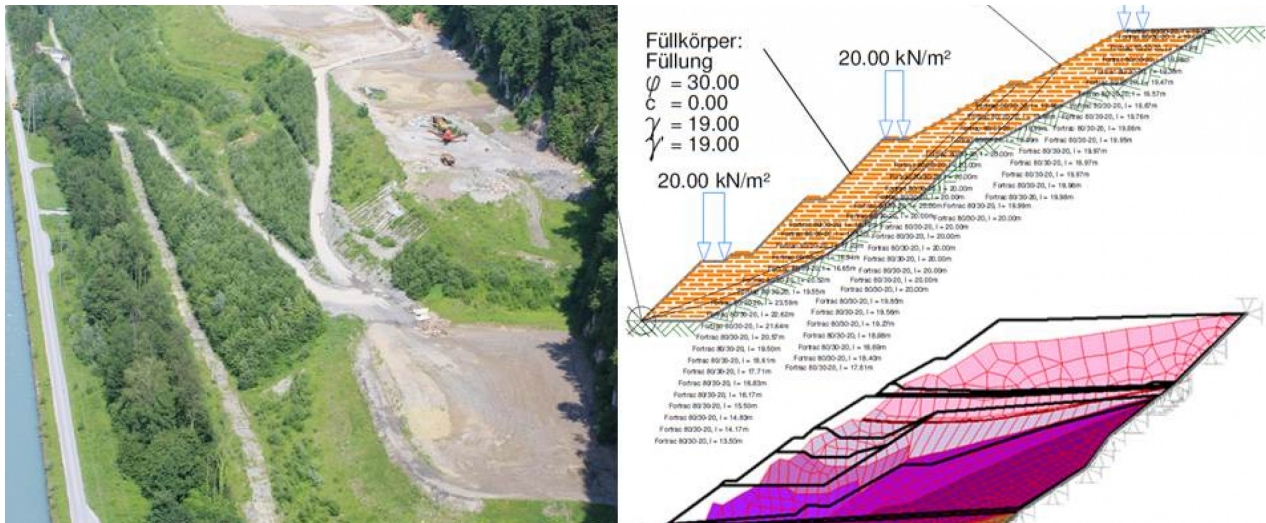
Deponie Gäsi und Ergebnisse der Deformations- und Stabilitätsberechnungen (Bilder: FRIEDLIPARTNER AG)
